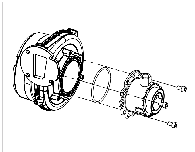
Obr. 27 Směšovač
