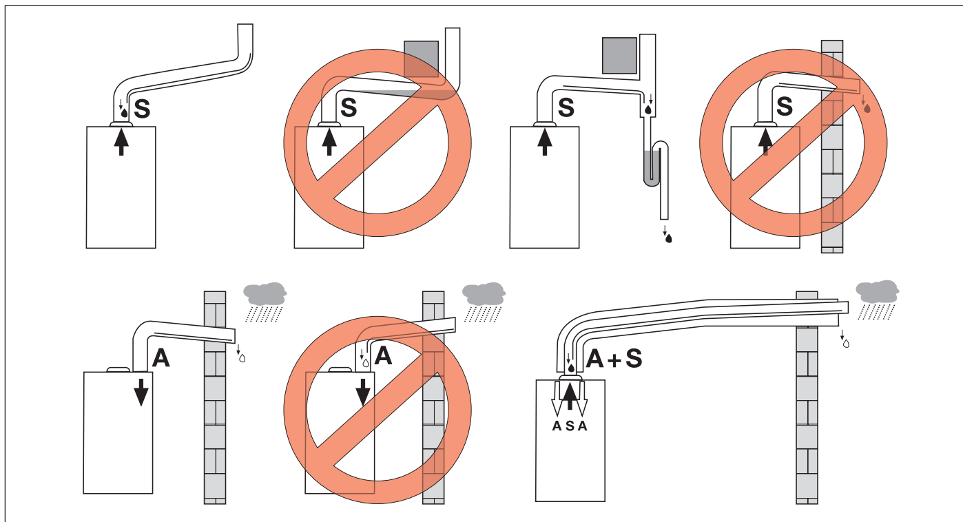
Obr. 10 Příklady instalace
