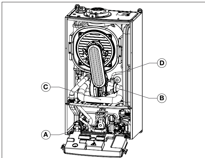
Obr. 26 Sací trubice
