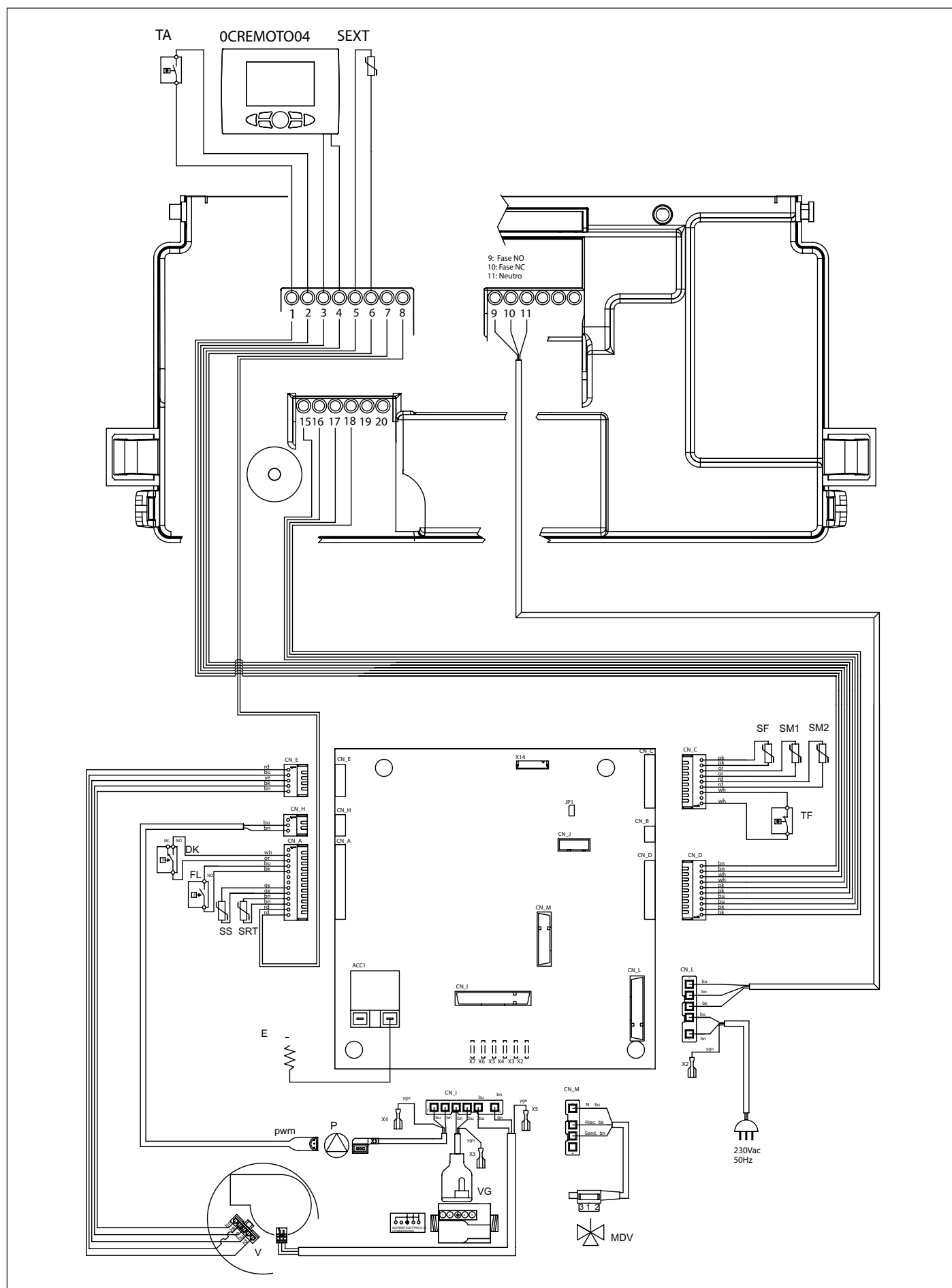
Obr. 23 Elektrické schéma KC
