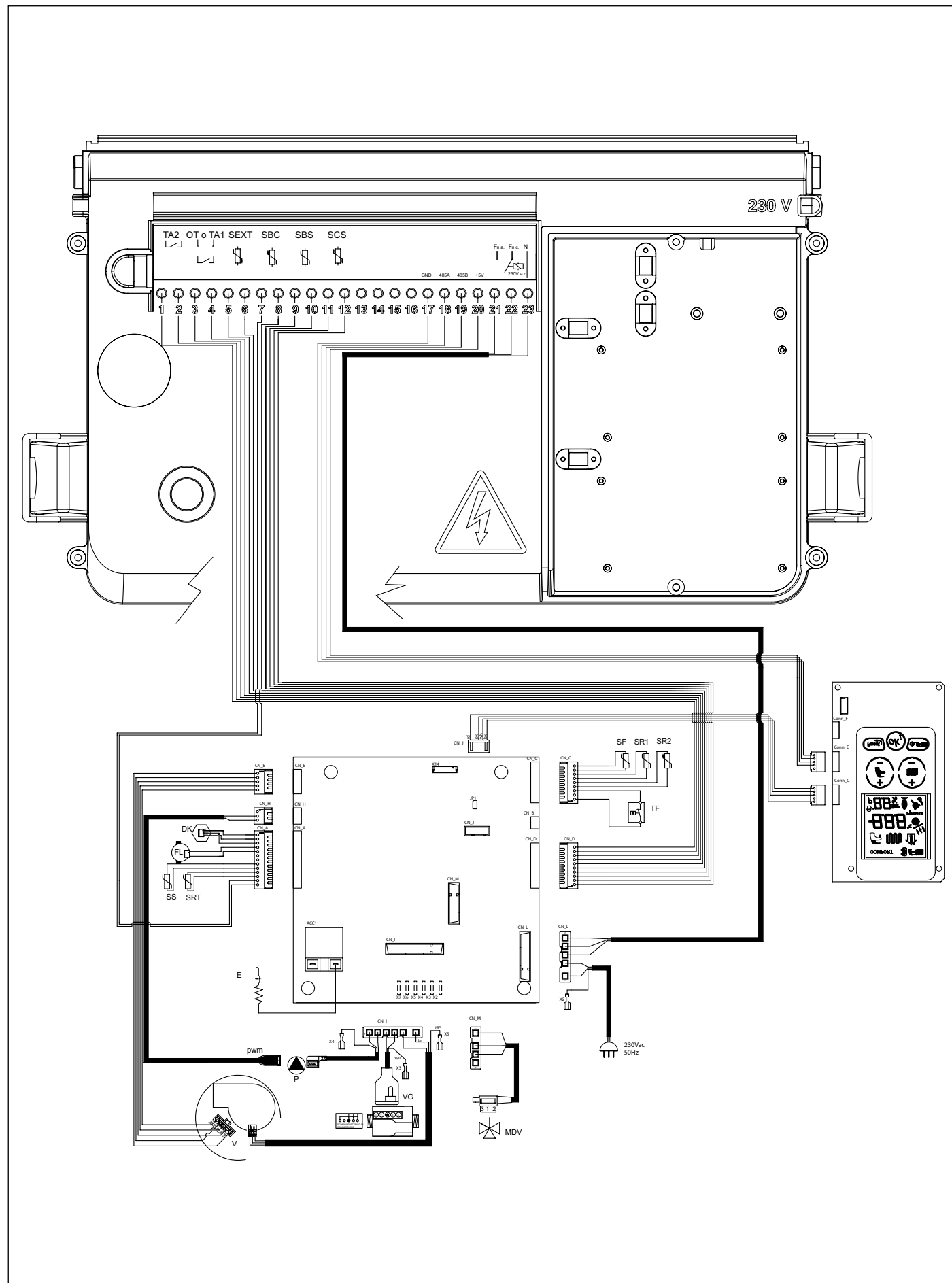
Obr. 24 Elektrické schéma KC
