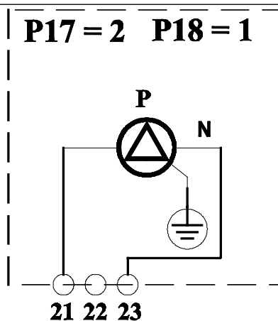
Obr. 25 Elektrické schéma solárního systému s nuceným oběhem a kombinovaným kotlem
