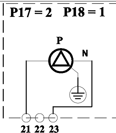
Obr. 30 Elektrické schéma solárního systému s nuceným oběhem a kotlem pouze pro ÚV
