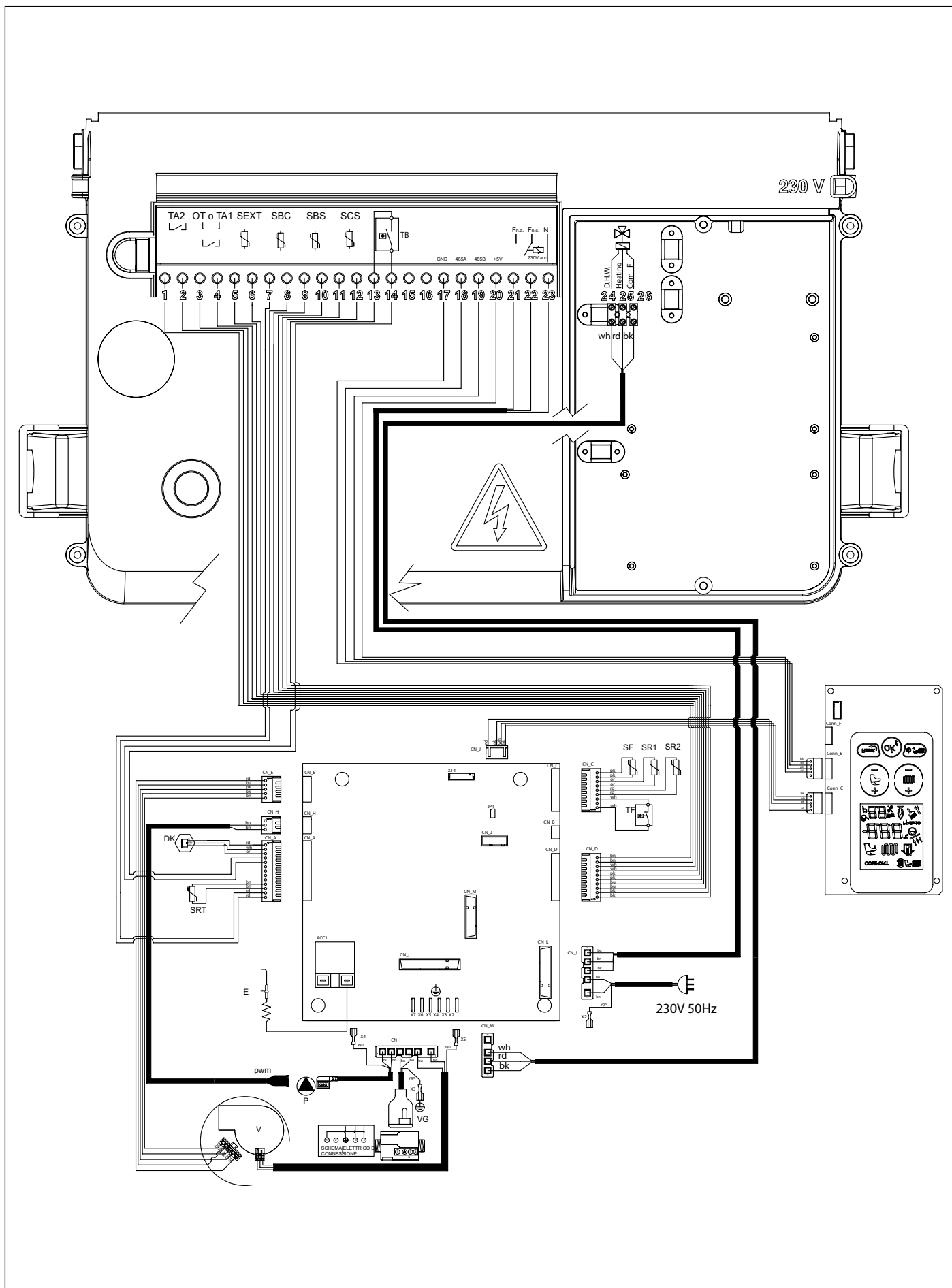
Obr. 29 Elektrické schéma model KR
