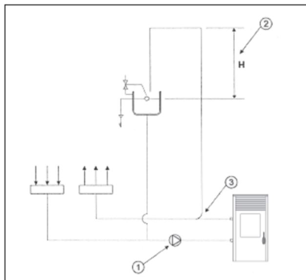
Diagram systému s otevřenou expanzní nádobou
