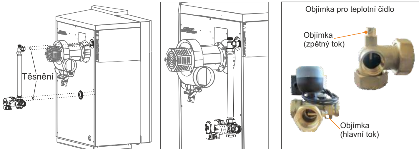
Příklad instalace skupina čerpadel do kotle PelTec II Lambda 18-36
