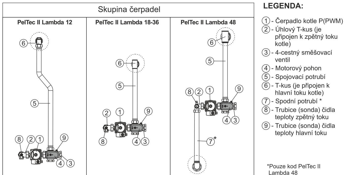
Příklad instalace skupina čerpadel do kotle PelTec II Lambda 18-36
