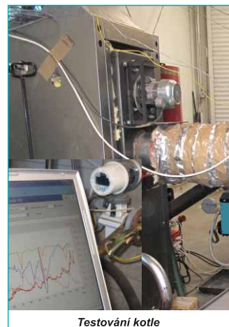
Testování kotle
