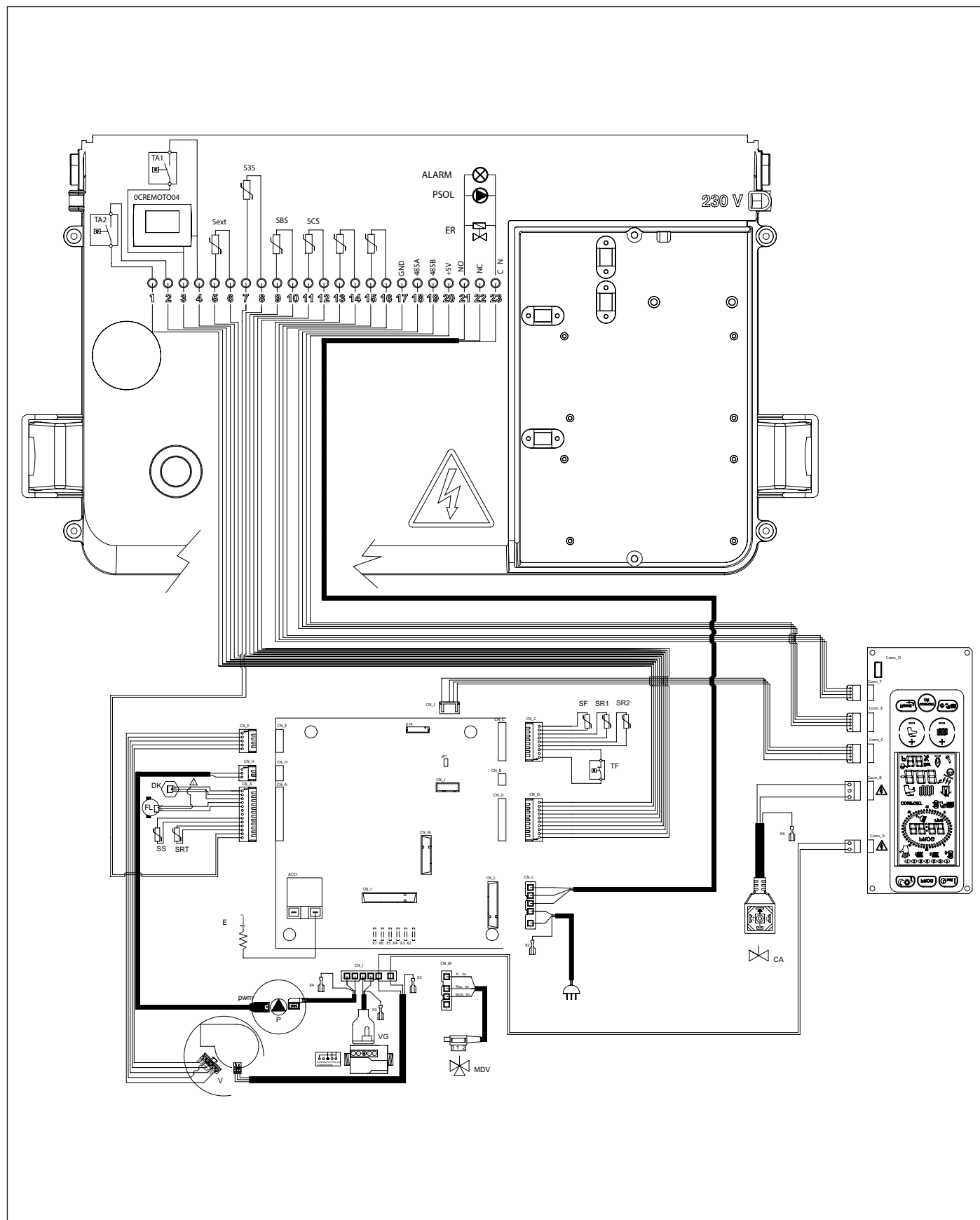
Obr. 24 Elektrické schéma KC
