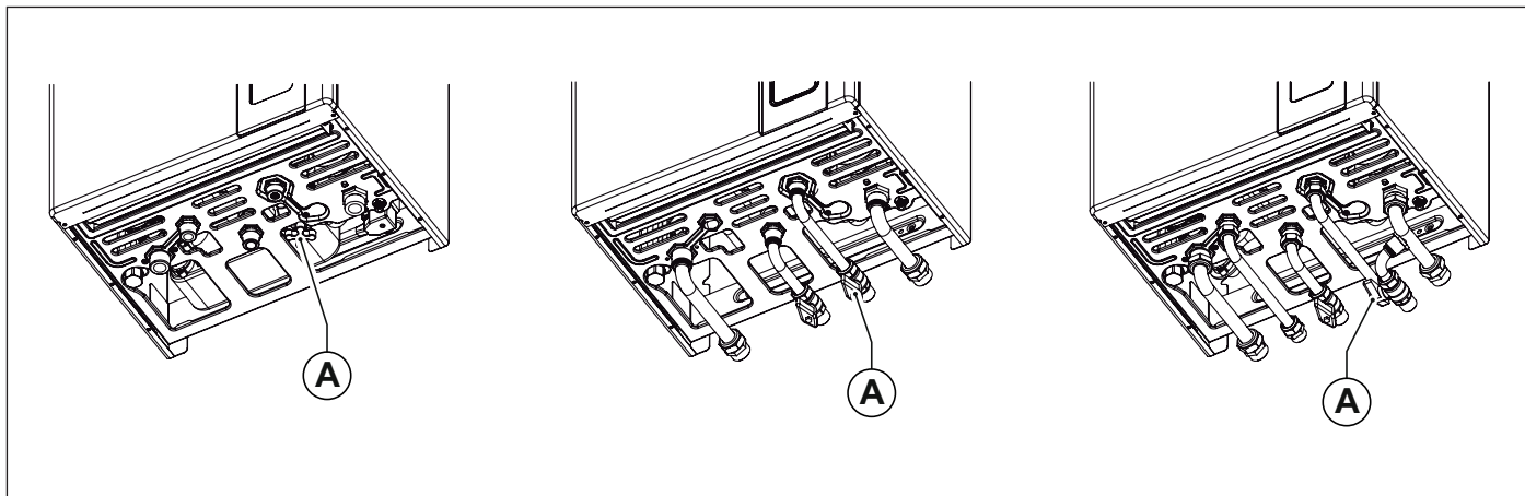
Obr. 2 Plnicí kohouty
