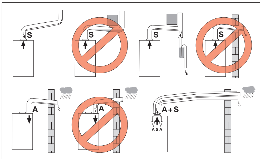
Obr. 10 Příklady instalace
