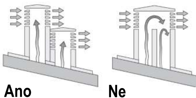
Obr. 5: Charakteristika komína
